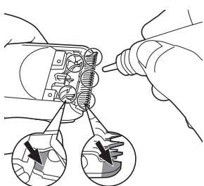
Lubrification en utilisant la plaque coulissante d'entretien
