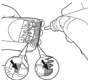
Smarowanie za pomocą wysuwanej płytki do celów konserwacji
