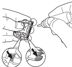
Lubrification avec les lames retirées
