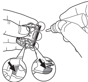
Smering met de messen verwijderd
