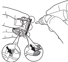
Smarowanie z wyjętymi ostrzami
