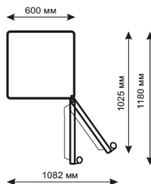
Рабочие габариты холодильного прибора.
