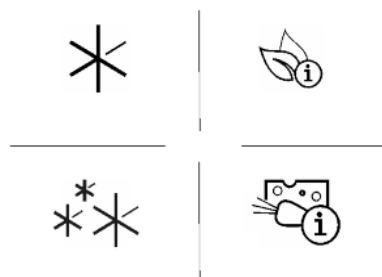
Fig. 10 Программные
