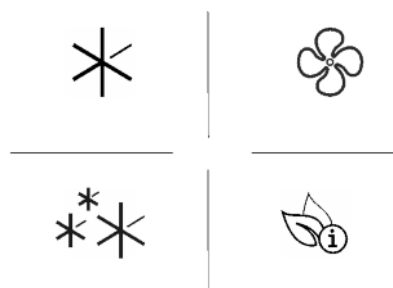
Fig. 9 Программные
