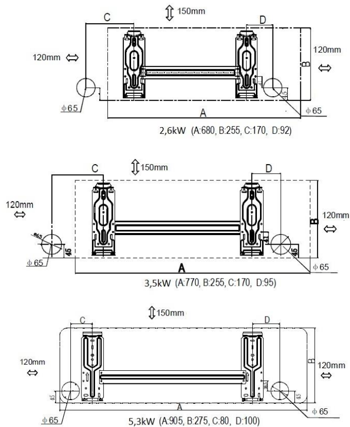
Slika 5: Priporočene pozicije lukenj za plinsko in električno povezavo
