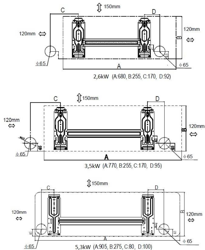
Slika 5. Preporučljivi položaji rupa za plinsko i električno povezivanje
