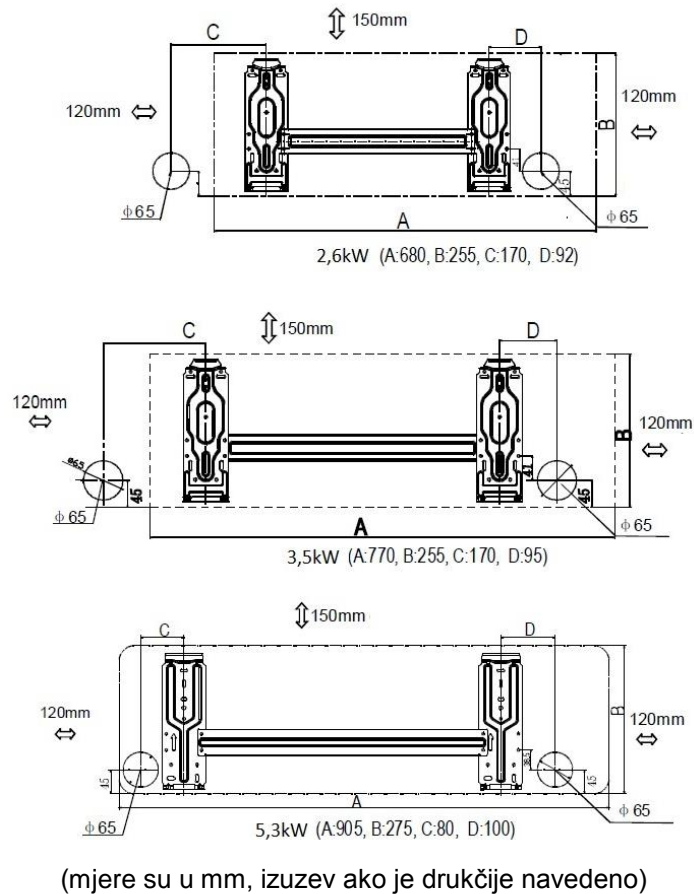
Slika 5. Preporučljivi položaji rupa za plinsko i električno povezivanje
