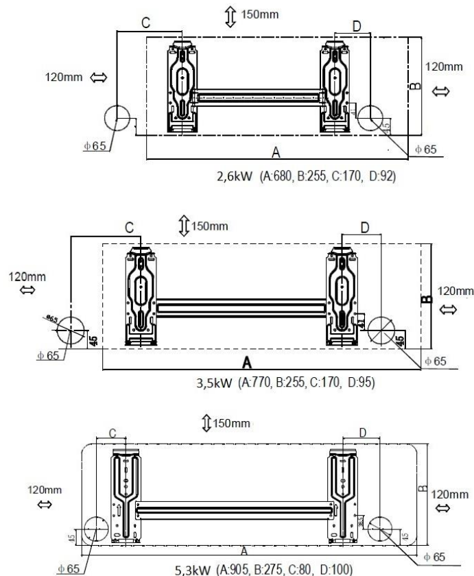
Слика 5. Препоручљиви положаји рупа за гасно и електрично повезивање
