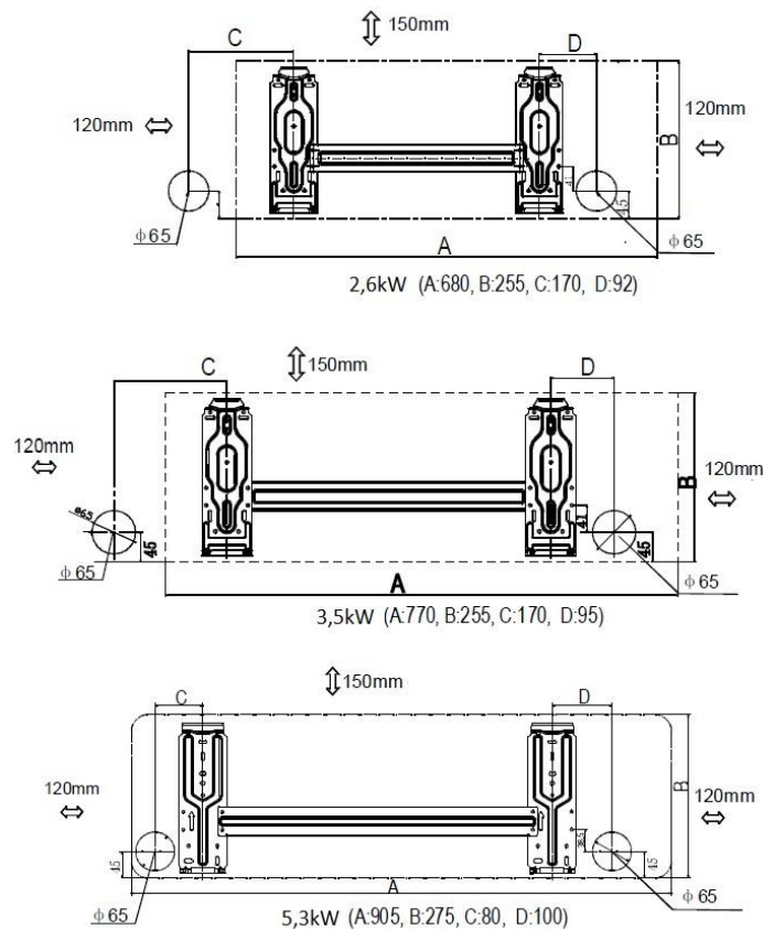
Slika 5. Preporučljivi položaji rupa za plinsko i električno
